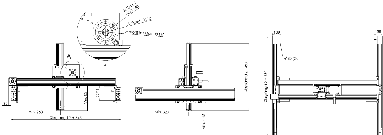
Mått på X-axelns drivaxelhus se linjärenhet ALR26. Mått på Y-axelns drivaxelhus se linjärenhet ALR23.
