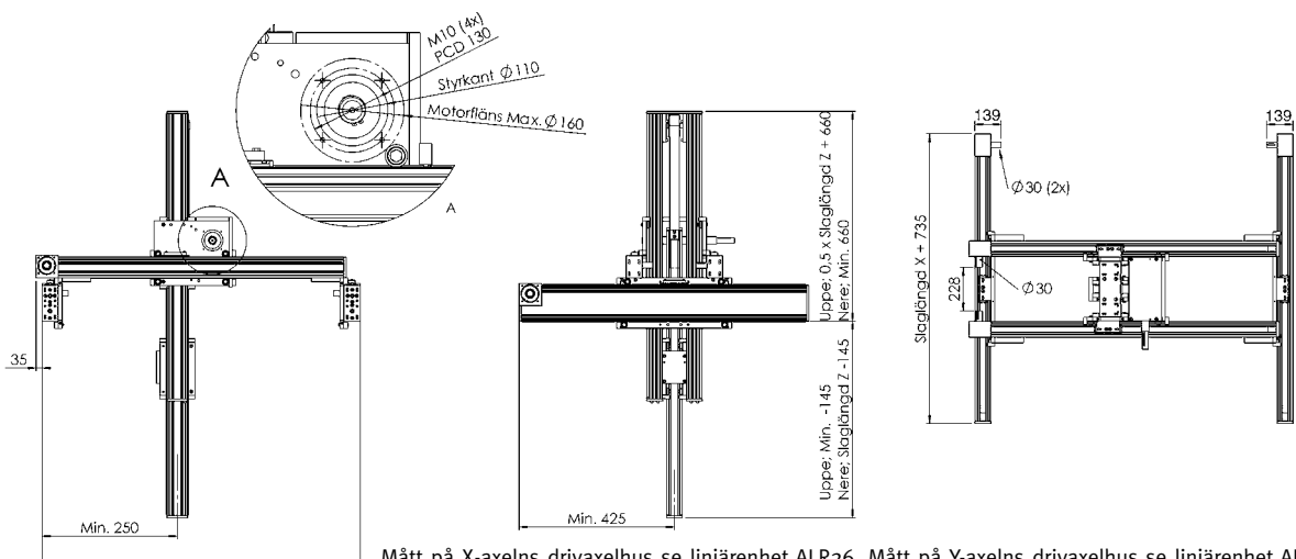
Mått på X-axelns drivaxelhus se linjärenhet ALR26. Mått på Y-axelns drivaxelhus se linjärenhet ALR23.
